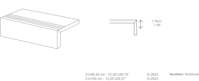
Step 45° 2cm | Step 45° 2cm
