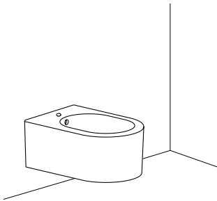
BIDET SOSPESO OTIS MONOFORO Otis wall-hung bidet with 1 hole cm 56 x 38,5 x 25 h
